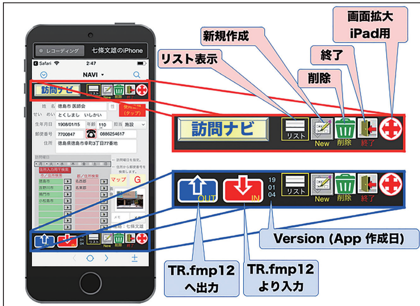
図 7 : 『訪問 NAVI』 の初期画面の説明 1
